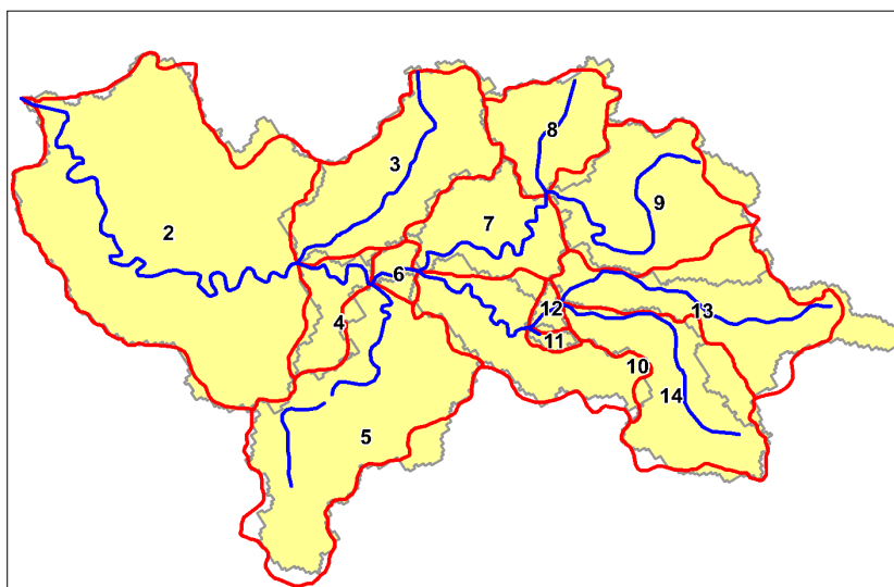
Рисунок 1. Соответствие бассейнов р.Тойтьёган, выделенных по топографической карте масштаба 1: 200 000 (красный цвет), а также на основе глобальной модели рельефа GMTED 2010 (желтый фон, черный цвет)
