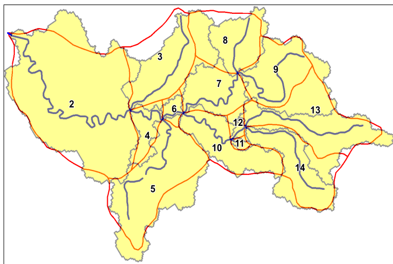
Рисунок 4. Соответствие границ бассейнов р.Тоитъёган, выделенных по топографической карте масштаба 1: 1 000 000 (красный цвет), а также на основе глобальной модели рельефа GMTED 2010 (желтый фон, черный цвет)
